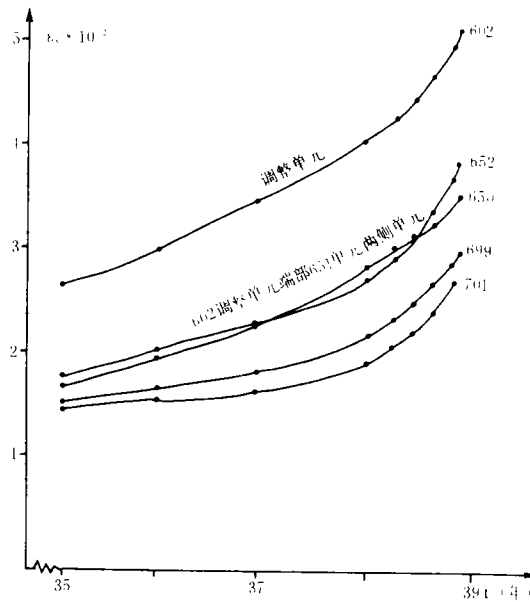
图8 模型I中调整单元602及其附近点的 \epsilon_x-t 曲线
